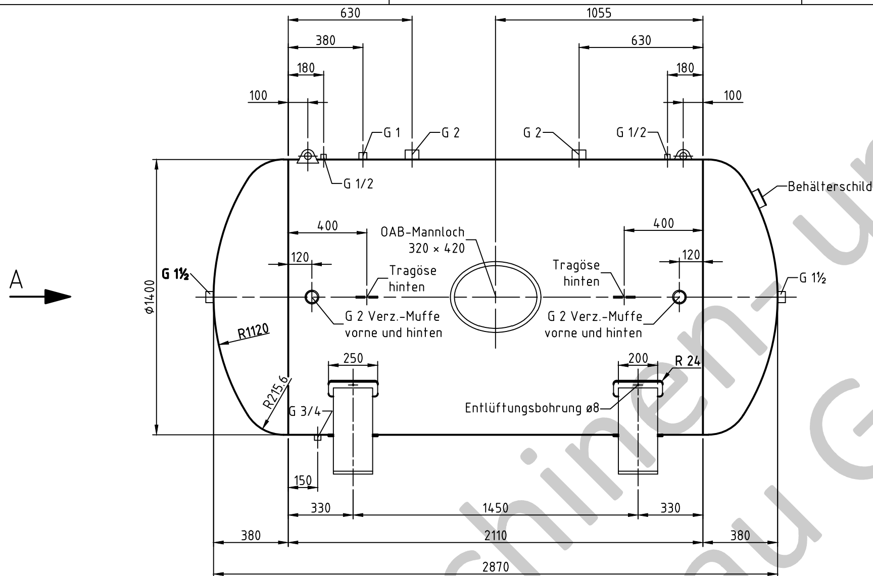
Ansicht A
